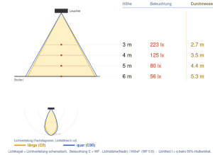
Ausleuchtung (Richtwert) 7050M6 - 15W 4000K (CRI > 90) - 1200 lm Halbwinkel 24° (Ang. 250°) - 24° (Ang. 250°)
