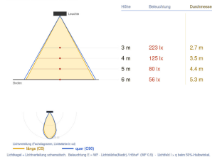
Ausleuchtung (Richtwert) 7050M6 - 15W/4000K/150° - 1200 lm Halbwinkel 24° (Ang. 0.5) / 24° (Ang. 0.5)
