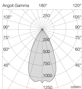
Ausleuchtung (Richtwert) 7050M6 - 15W/4000K/150° - 1200 lm Halbwinkel 24° (Ang. 0.5) / 24° (Ang. 0.5)
