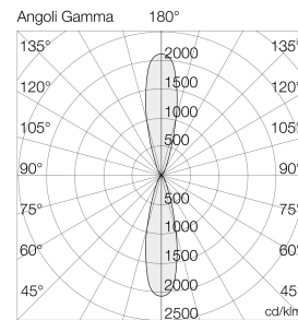
Ausleuchtung (Richtwert) 7054B3 - MAX 7054B3MILO - 1 - 2007-19 Höhenwerte 17' (5,18 m) - 17' (5,18 m)
