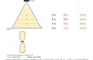
Ausleuchtung (Richtwert)
