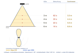
Ausleuchtung (Richtwert) 7054B6 - MAXI 19W/4000K/19 - 2000 lx Höhenwerte (20°-80°) (10°-135°) (10°-135°)
