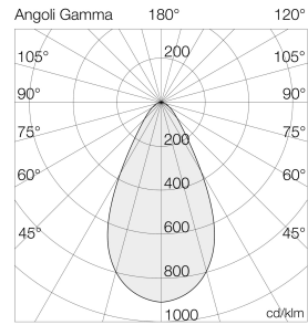
Ausleuchtung (Richtwert) 7054M6 - MILO (M6) 23W 3000K Anthrazit Höhenabstand 20° (10° - 30°) 100° (10° - 30°)
