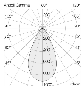
Ausleuchtung (Richtwert) 7055S6 - ARIS (S6) 20W 3000K Silber Höhenwerte 20° (100°) 100° (100°) 100° (100°)
