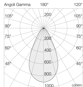
Ausleuchtung (Richtwert) 7055S6 - ARIS 10W/4000K/10 - 1000 lx Höhenwerte 27° (300 lx) / 30° (200 lx)
