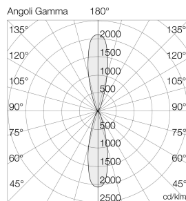
Ausleuchtung (Richtwert) 7056B33020SL - 1000 lm (3000K) - 20W Halbkegel 10° (Ang. 0.5) / 10° quer (0.5)
