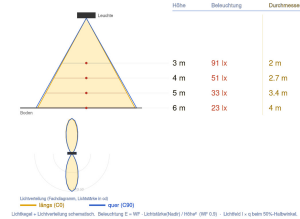
Ausleuchtung (Richtwert) 7056B33020SL - 1000 lm (3000K) - 20W Halbkegel 10° (Ang. 0.5) / 10° quer (0.5)
