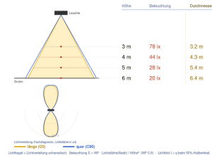
Ausleuchtung (Richtwert) 7056B6 - 1000 7056B6/30W 3000K 60° Halbwinkel (20°) (30°) (40°) (50°) (60°)
