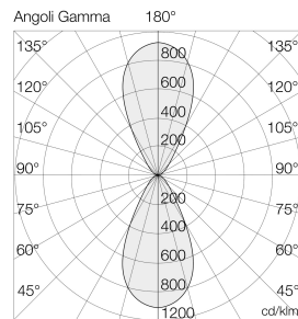
Ausleuchtung (Richtwert) 7056B6 - 1000 7056B6/30W 3000K 60° Halbwinkel (20°) (30°) (40°) (50°) (60°)
