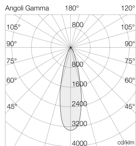
Ausleuchtung (Richtwert) 7056M33020BD - 162x162x162mm - 20W 3000K Halbwinkel 10° (Ang. 0.33°) / 10° (Ang. 0.33°)
