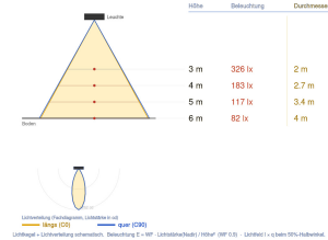
Ausleuchtung (Richtwert) 7056M33020BD - 162x162x162mm - 20W 3000K Halbwinkel 10° (Ang. 0.33°) / 10° (Ang. 0.33°)
