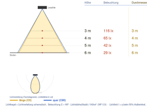
Ausleuchtung (Richtwert) 7056M6 - M6 (3000K) 10W 3000K Halbwinkel 27° (Ang. 0.5) 20° (Ang. 0.3)
