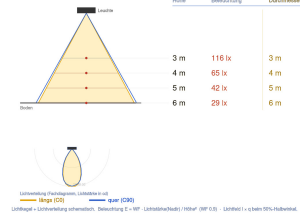
Ausleuchtung (Richtwert) 7056M6 - 10W/3000K/30° - 120°/162
