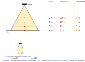
Ausleuchtung (Richtwert) 2056M6 - M63020CL - 2000 lx Halbwinkel 27° (Ang. 0.5) - 28° (Ang. 0.5)
