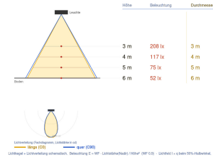
Ausleuchtung (Richtwert) 2056M6 - M63020GD - 20W 3000K Halbwinkel 27° (Ang. 0.5) / 28° (Ang. 0.5)
