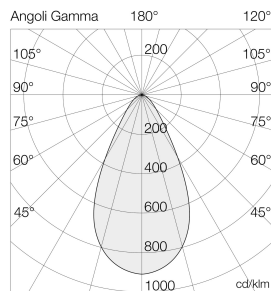
Ausleuchtung (Richtwert) 7056M6 - M63020SD - 2000 lx Halbwinkel 27° (Ang. 0.5) - 20° (Ang. 0.3)
