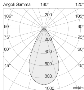
Ausleuchtung (Richtwert) 7056M6 - M63030GD - 30W 3000K Halbwinkel 27° (Ang. 0.5) / 27° (Ang. 0.5)
