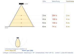
Ausleuchtung (Richtwert) 7056M6 - M63030SD - 30W 3000K Halbwinkel 27° (Ang. 0.5) - 20° (Ang. 0.3)
