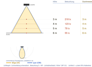
Ausleuchtung (Richtwert) 7056M6 - M6 (20W/4000K) - 1200 lx Halbwinkel 27° (Ang. 0.5) - 20° (Ang. 0.25)
