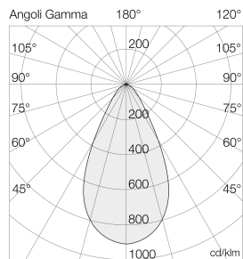
Ausleuchtung (Richtwert) 7056M6 - M6 (30W/4000K) - 1200 lx Halbkegel 27° (Ang. 0.5) - 20° (Ang. 0.35)
