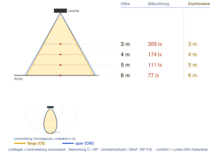
Ausleuchtung (Richtwert) 7056M6 - M6 (30W/4000K) - 1200 lx Halbkegel 27° (Ang. 0.5) - 20° (Ang. 0.35)
