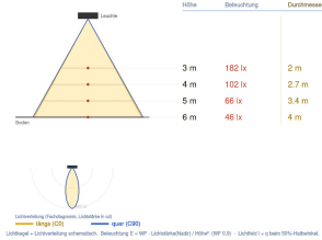
Ausleuchtung (Richtwert) 7056S3 - 10W 3000K S3 - 1175 lx Halbwinkel 10° (Ang. 0.5) 10° (Ang. 0.5)
