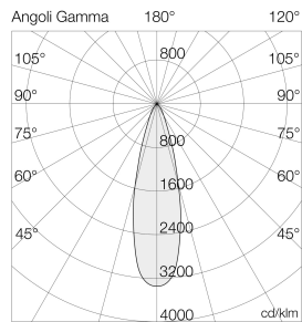
Ausleuchtung (Richtwert) 7056S3 - 10W 3000K S3 - 1175 lx Halbwinkel 10° (Ang. 0.5) 10° (Ang. 0.5)
