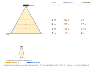
Ausleuchtung (Richtwert) 7056S3 - MAX 7056S3(S3) - 2019-19 Halbwinkel 10° (Angl. 0.17) 10° (Angl. 0.17)
