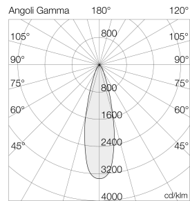
Ausleuchtung (Richtwert) 7056S3 - MAX 7056S3(S3) - 2019-19 Halbwinkel 10° (Angl. 0.17) 10° (Angl. 0.17)
