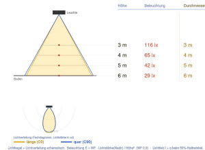
Ausleuchtung (Richtwert) 7056S6 - 10W 3000K (S6) - 1200 lx Halbwinkel 27° (Ang. 0.5) - 20° (Ang. 0.5)
