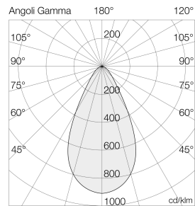
Ausleuchtung (Richtwert) 7056S6 - 10W 3000K (S6) - 1200 lx Halbwinkel 27° (Ang. 0.5) - 20° (Ang. 0.5)
