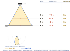
Ausleuchtung (Richtwert) 7056S6 - 10W 3000K/10 - 1200 lx Halbwinkel 27° (Ang. 0.5) - 20° (Ang. 0.3)
