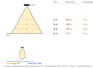
Ausleuchtung (Richtwert) 7056S6 - 1000 7056S6/30W 1 3000 K Halbwinkel 27° (Ang. 0.5) (BSP. 0.5m)
