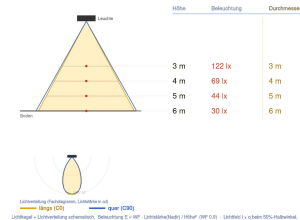
Ausleuchtung (Richtwert) 7056S6 - 10W 4000K (S6) - 1.000 lx Halbwinkel 27° (Ang. 0.5) - 0.5° (Ang. 0.5)
