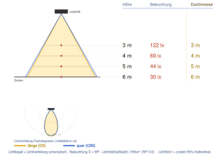
Ausleuchtung (Richtwert) 7056S6 - 10W 4000K (S6) - 1.000 lx Halbwinkel 27° (Ang. 0.5) - 20° (Ang. 0.3)
