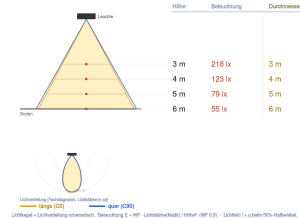
Ausleuchtung (Richtwert) 7056S6 - 10W 2000K/4000K - 1200lm Halbwinkel 27° (Ang. 0.5) - 20° (Ang. 0.3)
