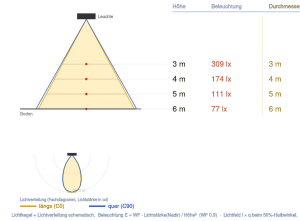
Ausleuchtung (Richtwert) 7056S6 - 1000 1000x1000 - 1000 lx Halbwinkel 27° (Ang. 0.5) - 20° (Ang. 0.5)
