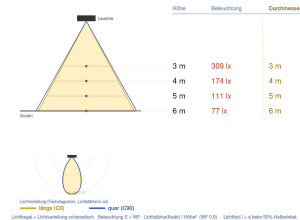
Ausleuchtung (Richtwert) 7056S6 - 1000 1000x1000 - 1 1000 lx Halbwinkel 27° (Ang. 0.5) - 0.5° (Ang. 0.5)
