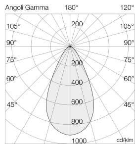
Ausleuchtung (Richtwert) 7056S6 - 1000 lx (1000 lx) - 1000 lx Halbwinkel 27° (Ang. 0.5) - 27° (Ang. 0.5)
