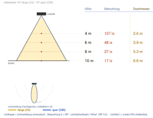
Ausleuchtung (Richtwert) 7155V2 - MAN 7106V2M990 - 1 61801 (m)
