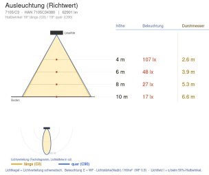
Ausleuchtung (Richtwert) 7155V2 - MAN 7106V2M990 - 1.65001 km
