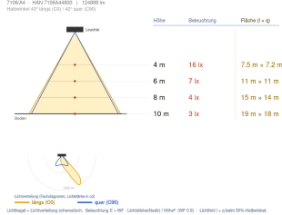
Ausleuchtung (Richtwert)
