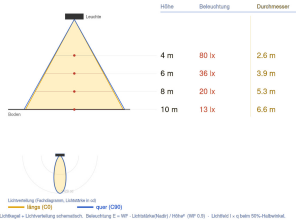
Ausleuchtung (Richtwert) 7106/C3 - HAN 7106C34060 | 152238 lm Halbwinkel 18° längs (C0) / 19° quer (C90)
