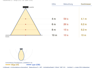
Ausleuchtung (Richtwert)
