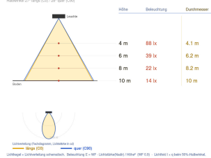
Ausleuchtung (Richtwert)
