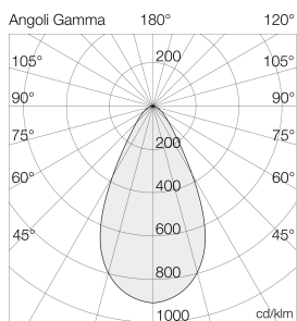
Ausleuchtung (Richtwert) 7112MR4500GL - 500W 4000K CRI 70 Halbkegel 20° (Höhe 0,30m) - 20° (Höhe 0,30m)
