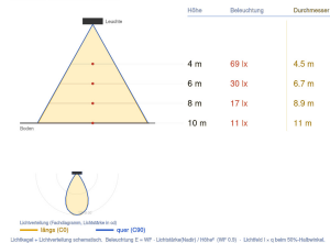
Ausleuchtung (Richtwert) 7112MR4500GL - 500W 4000K CRI 70 Halbkegel 20° (Höhe 0,30m) - 20° (Höhe 0,30m)
