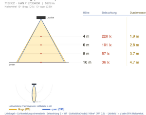
Ausleuchtung (Richtwert)
