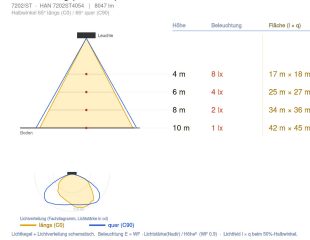
Ausleuchtung (Richtwert)
