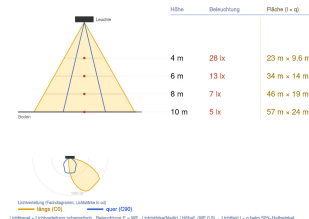
Ausleuchtung (Richtwert) 8029RR - 1000 mm (3000K) - 50W (3000K) - asymmetrische Optik
