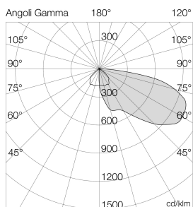
Ausleuchtung (Richtwert) 8029RR - 1000 mm (3000K) - 50W (3000K) - asymmetrische Optik
