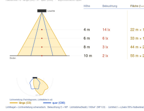
Ausleuchtung (Richtwert)
