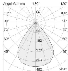
Ausleuchtung (Richtwert) 8150/52 - HAN 8150624770 | 13249 lm Halbwinkel 40° lings (C8) / 42° quer (C9C)
