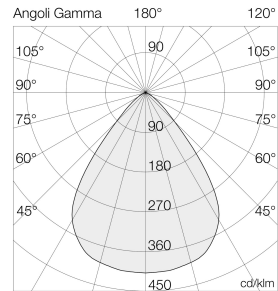
Ausleuchtung (Richtwert) 8150/S2 - HAN 8150/624110 | 20140 lm Halbwinkel 40° längs (D3) / 42° quer (D90)
