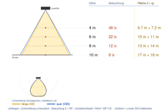
Ausleuchtung (Richtwert) 8150S2 - max 8150S24140 - 20700 lx Hallenstrahler 40° Strahl (11° - 14°) 140W (S2)
