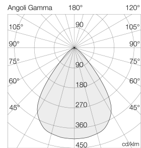
Ausleuchtung (Richtwert) 8150/S2 - HAN 8150G24170 | 30429 lm Halbwinkel 40° (längs) / 42° (quer) (C90)
