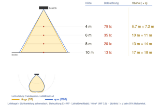
Ausleuchtung (Richtwert) 8150/S2 - HAN 8150/624245 | 40397 lm Halbwinkel 40° längs (D3) / 42° quer (D90)
