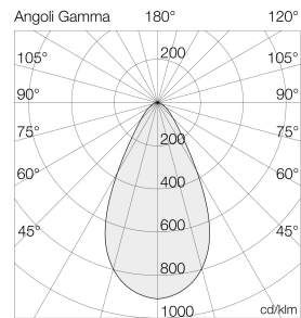
Ausleuchtung (Richtwert) 831I S2 - max 831I S2 (S2) 150W 4000K Silber Höhenabstand 30° (S2) 150W 4000K Silber
