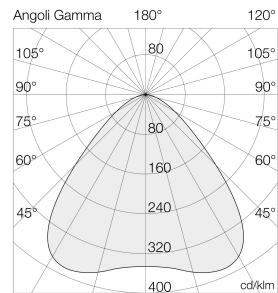
Ausleuchtung (Richtwert) 831IS54150G3 - 150W 4000K Silber Flächenleuchte 40° Strahlwinkel (10° - 40° Strahlwinkel)
