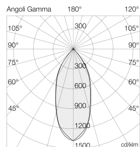
Ausleuchtung (Richtwert) 8400CU - Raum 8400CU4080GL - 10000 lm Hallenstrahler 20° (typ) (CU) 100° (typ) (CU)
